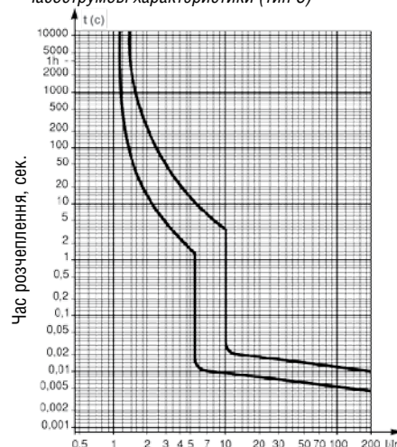
Часо-струмові характеристики (тип C)
